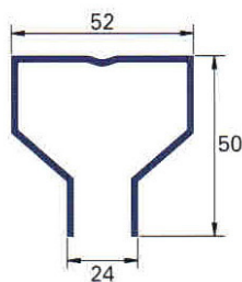
Perfil Bastidor
