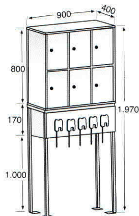
3 CSV2P + 1 MA900
