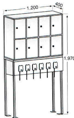
4 CSVS2P + 1 MA1200
